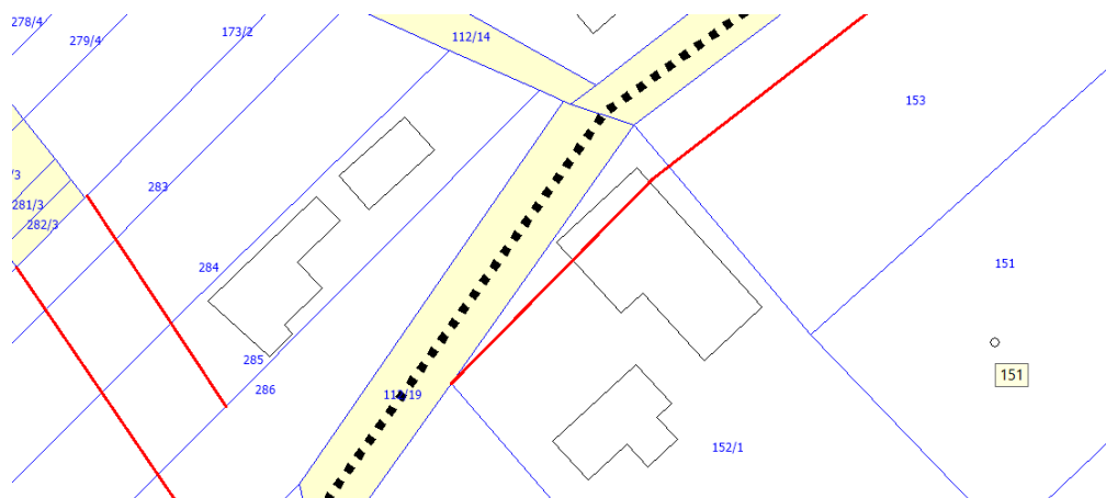
21. ábra – A 152/1 hrsz.-ú ingatlant érintő meglévő szabályozás (saját ábra)
