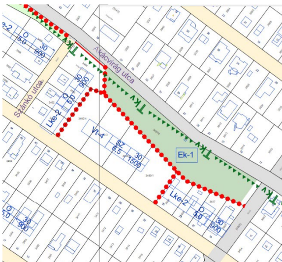
47. ábra - Hatályos Szabályozási terv részlet
