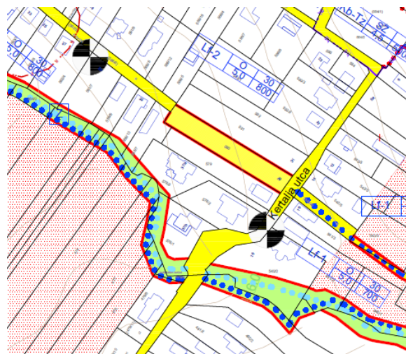
10. ábra - Javasolt Szabályozási terv részlet (saját ábra)
