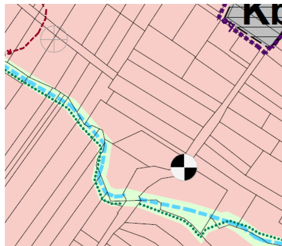
8. ábra - Hatályos Településszerkezeti terv részlet
