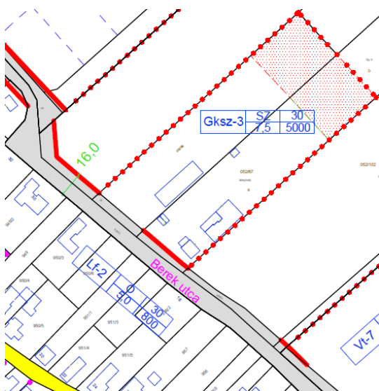
31. ábra - Hatályos Szabályozási terv részlet
