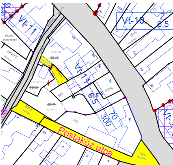
36. ábra - Hatályos Szabályozási terv részlet
