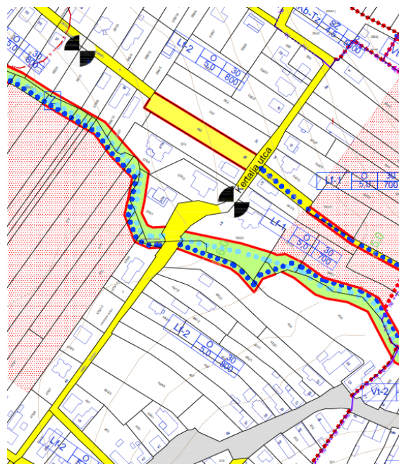
6. ábra - Javasolt Szabályozási terv részlet (saját ábra)
