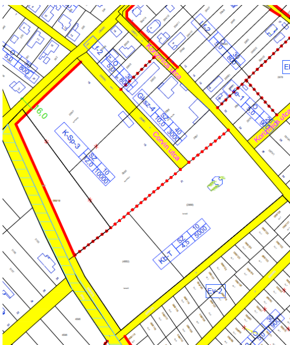
43. ábra - Hatályos Szabályozási terv részlet
