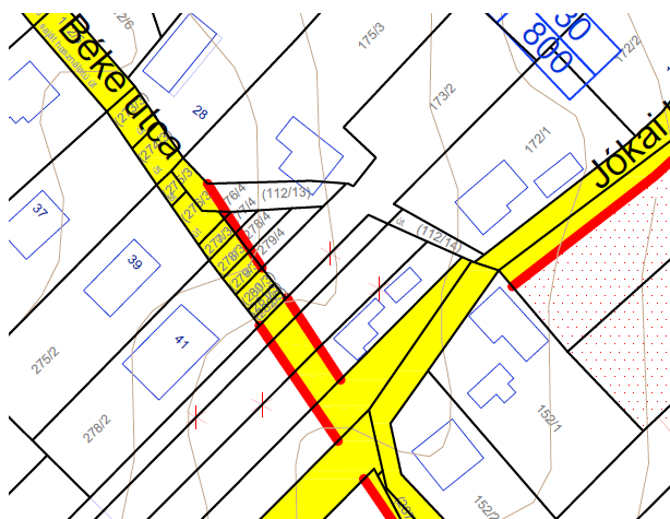
25. ábra - Javasolt Szabályozási terv részlet (saját ábra)
