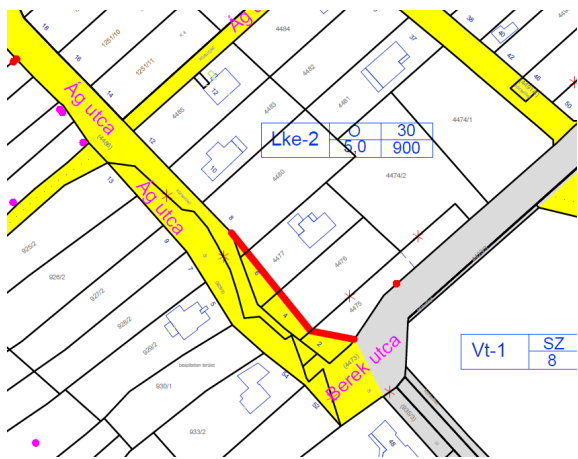
14. ábra - Hatályos Szabályozási terv részlet
