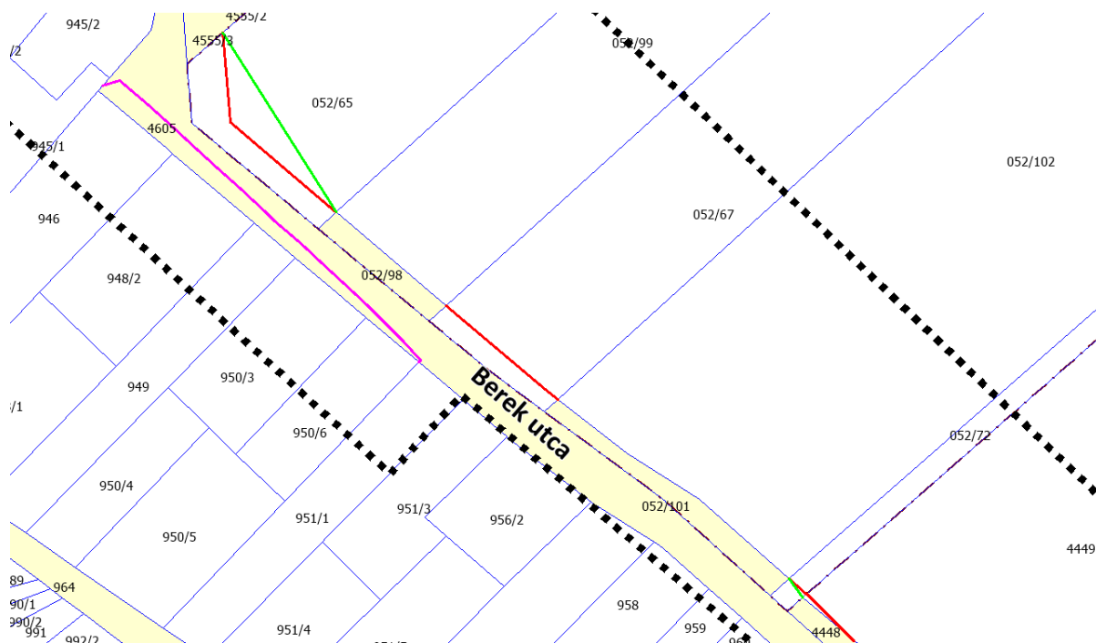
22. ábra - A meglévő és tervezett szabályozási vonalak, valamint a kerítések helyzete (A FEFTERV Kft. kiviteli terve alapján készült saját ábra)
