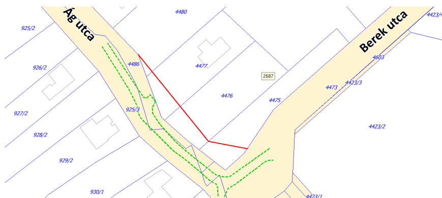
7. ábra - A szabályozási vonal és az útpálya helyzete (A FEFTERV Kft. kiviteli terve alapján készült (saját ábra)
