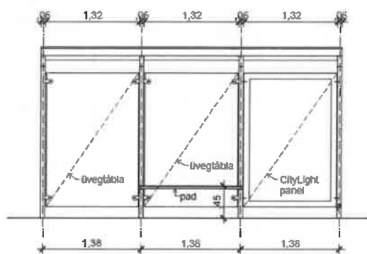
ELÖLNÉZET
