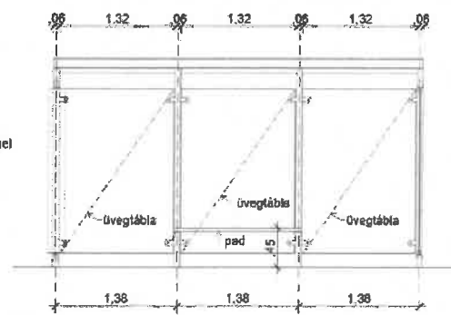
ELÖLNÉZET
